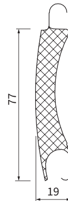
doorsnede lamel
