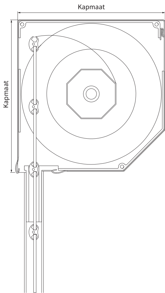
doorsnede kap
